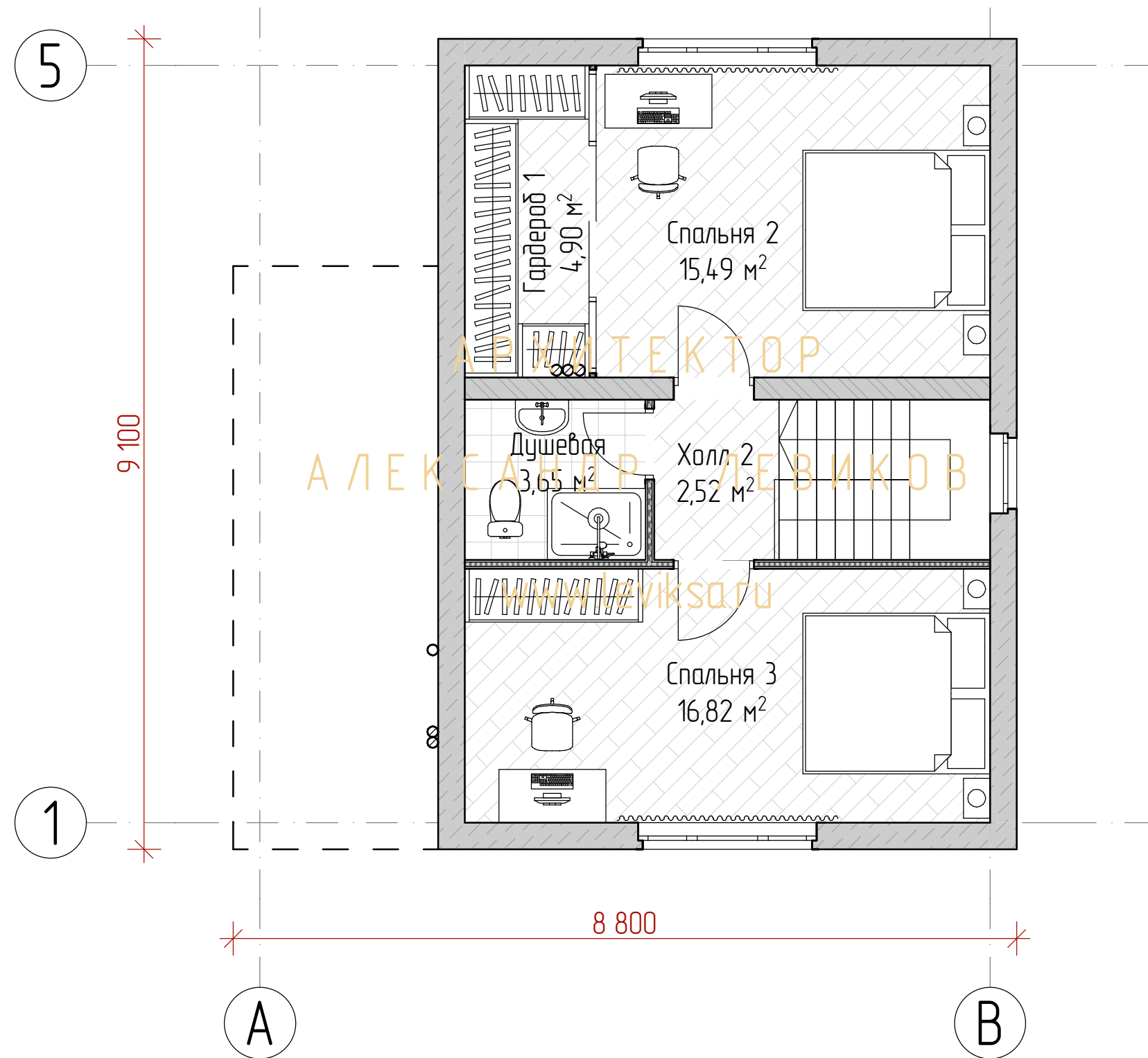
Экспликация помещений 2-го этажа
